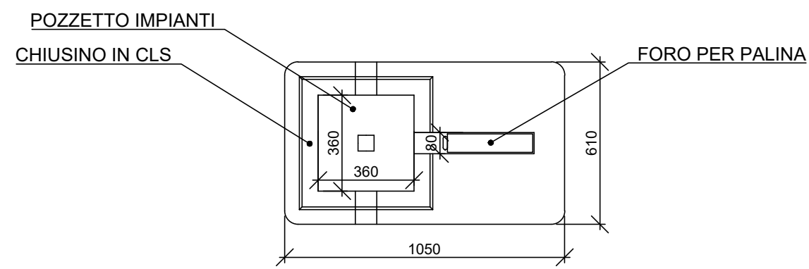
PIANTA PLINTO PER PALINA
